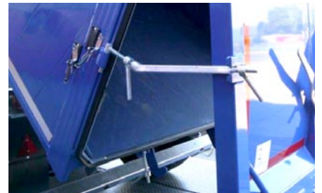
Abstandshalterung Heckklappe
